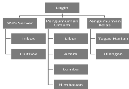
Gambar 8. Hirarki aplikasi
